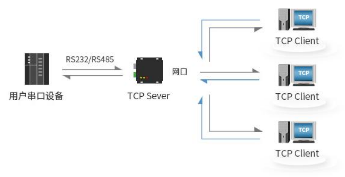
图 4-2 TCP Server
