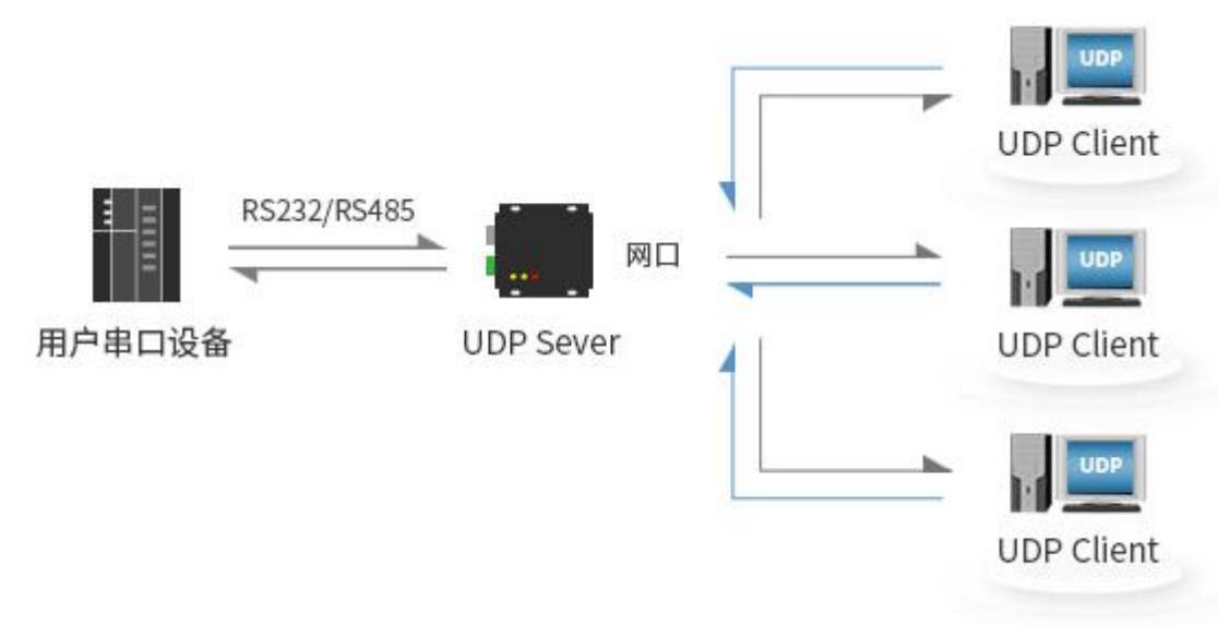
图 4-4 UDP Server
