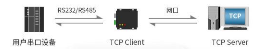
图 4-3 TCP Client
